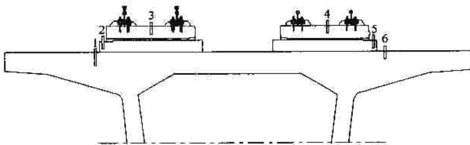
图 11.2.2—1 桥梁地段监测断面测点布设位置示意图
