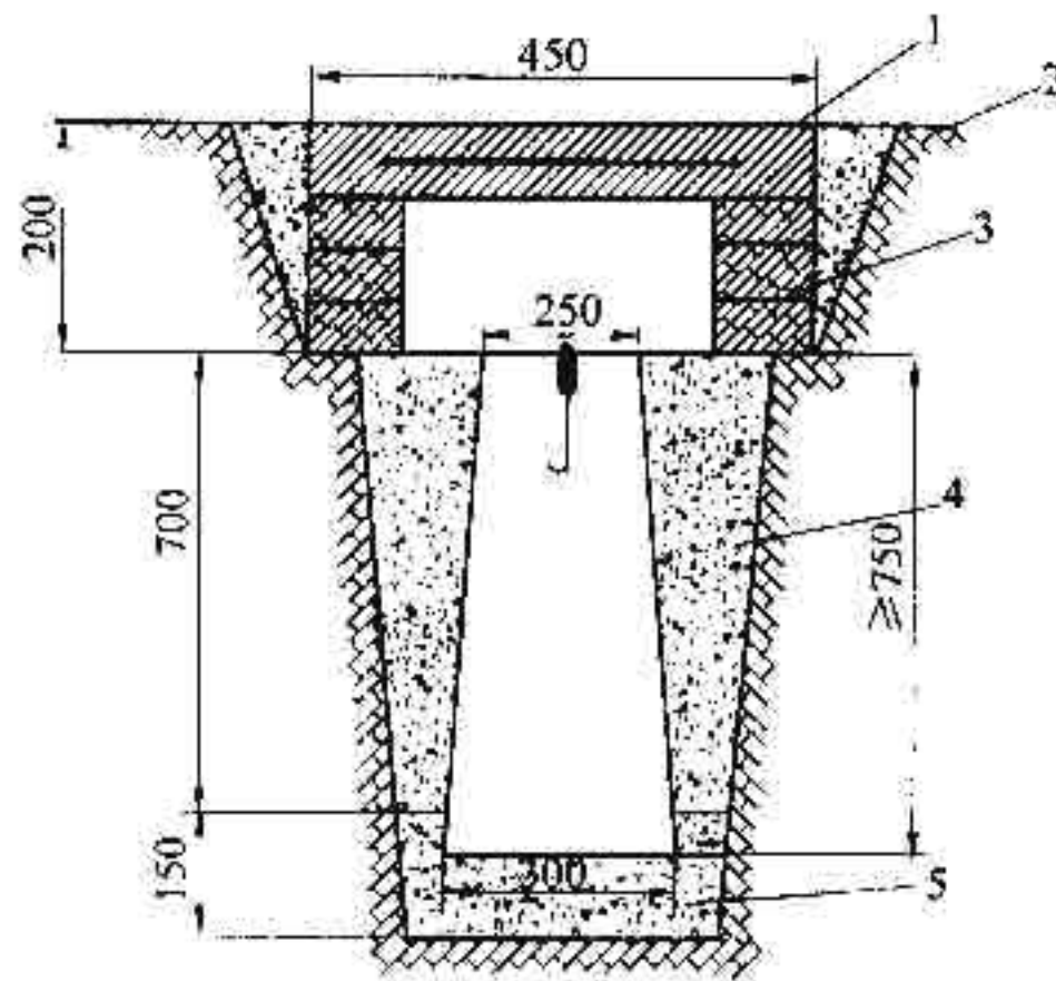
图 A. 2. 3 CP I 及二等平面控制点标石埋设图 (单位: mm)
