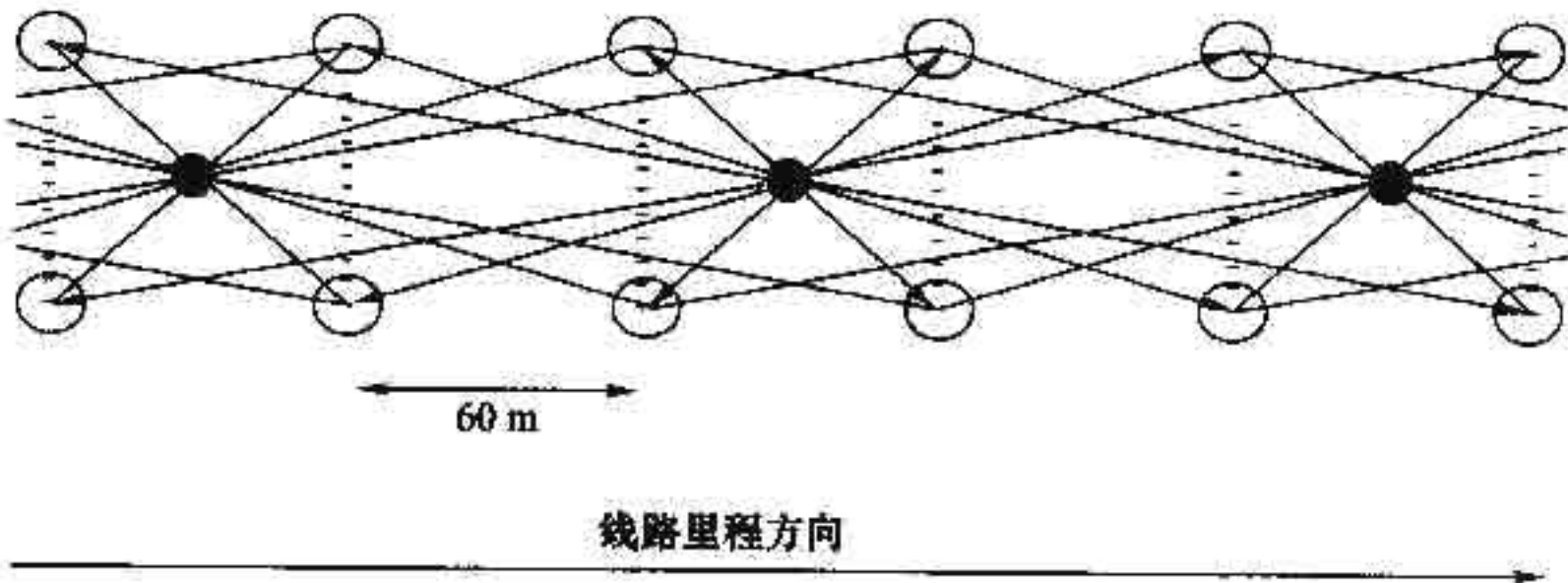
自由测站、CP III 点编号示意图
